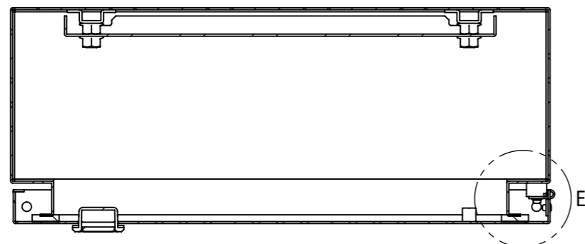
断面図 B-B
