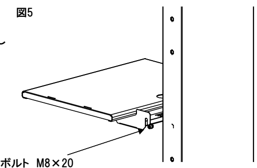
六角穴付ボルト M8×20
