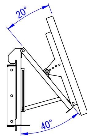
メンテナンス機構 (20° チルト、展開)
