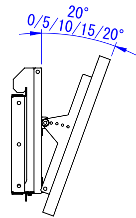
チルト詳細
