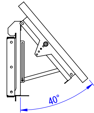
メンテナンス機構(展開)
