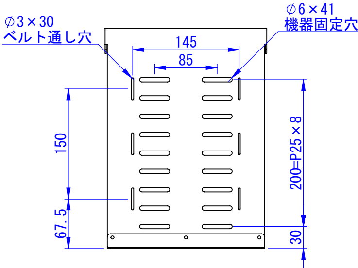
STB金具詳細 スケール 1:5
