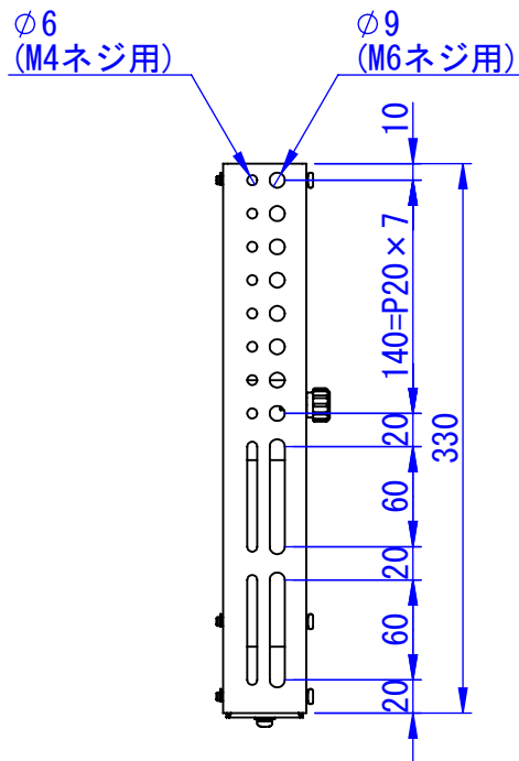
ディスプレイ取付金具詳細 スケール 1:5
