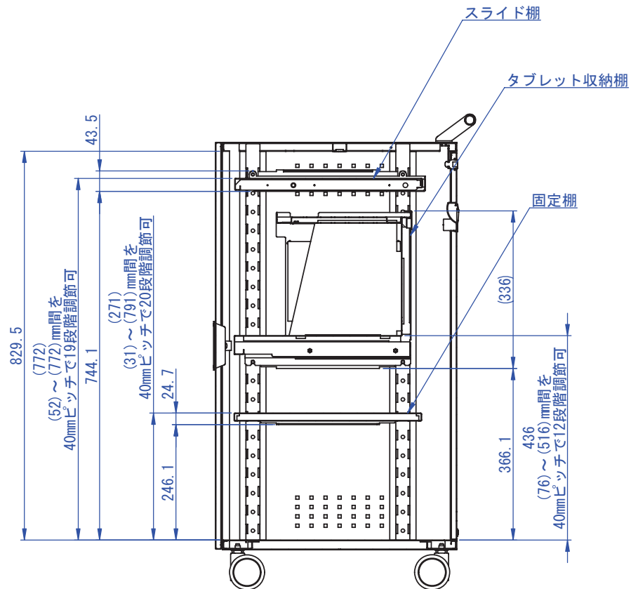
断面図 A-A
