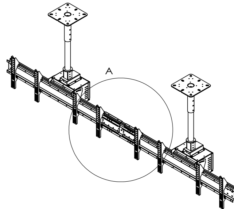
天吊り連結フレーム 取付イメージ
