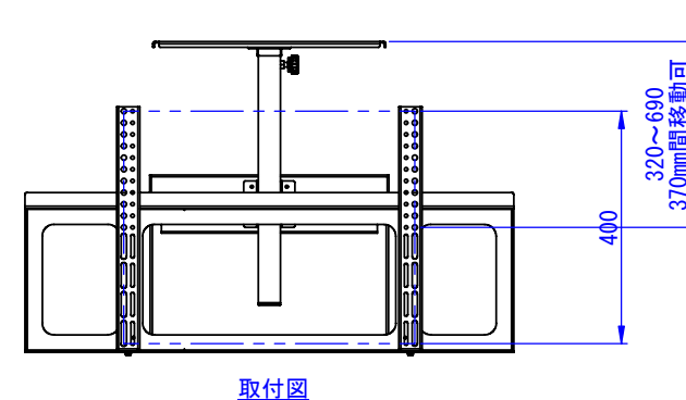
取付図
