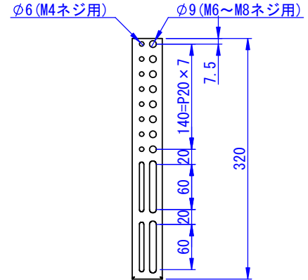
ディスプレイ取付金具詳細
