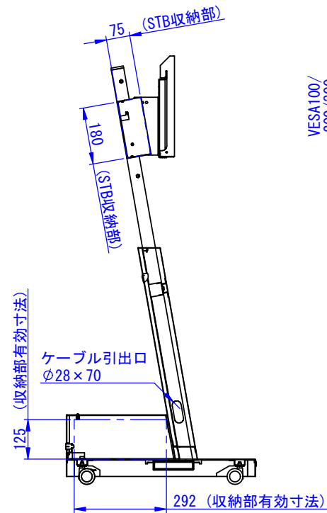
断面図 A-A
