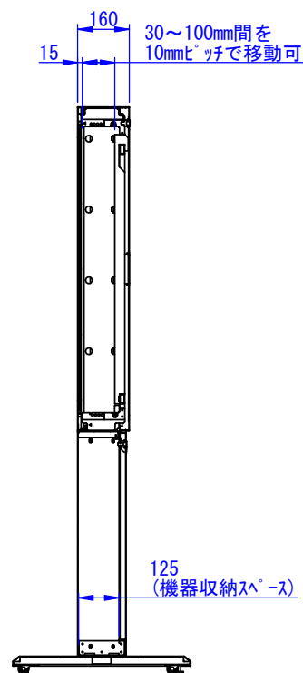
断面图 A-A
