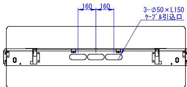
断面图 B-B
