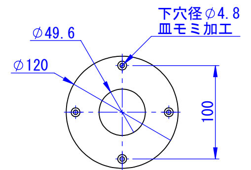
化粧板詳細
