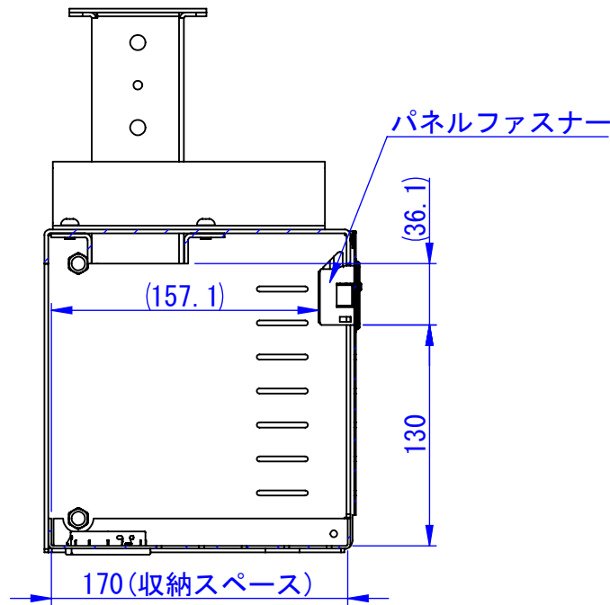
断面図 A-A
