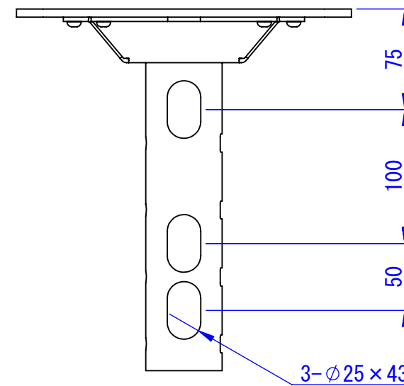
ベース詳細
