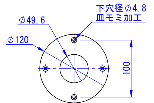
化粧板詳細
