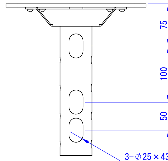
ベース詳細
