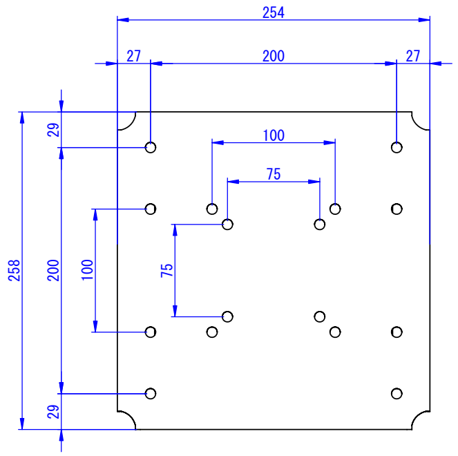
マウントプレート詳細 【VESA取付ピッチ】
