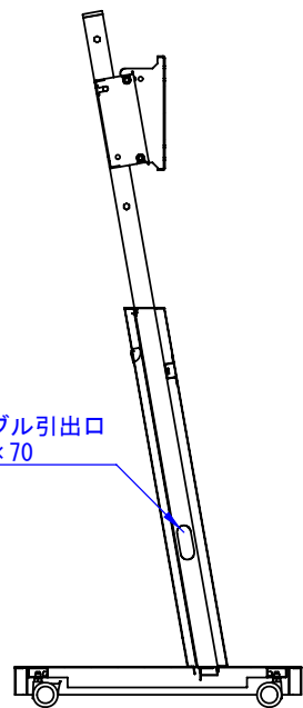
断面図 A-A
